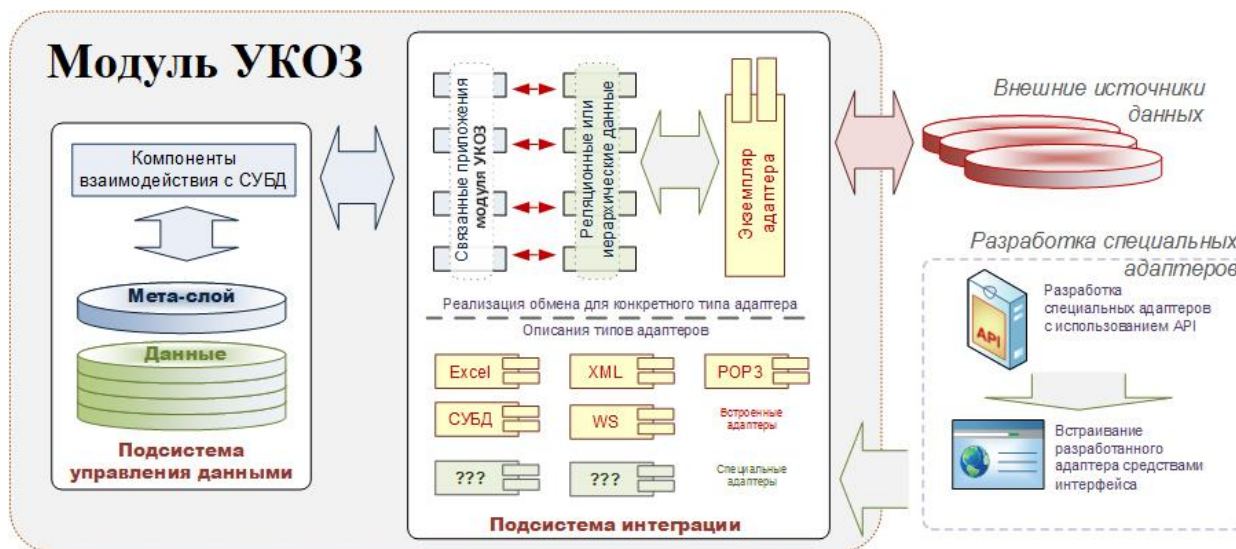
Рис. 1. Функциональная схема адаптера
